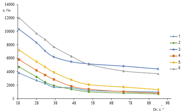
Рис. 2. Залежність структурної в'язкості модельних зразків від швидкості зсуву ( D_r ) за температури 20°C
