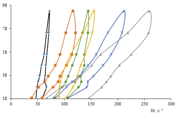
Рис. 1. Реограма залежності напруги зсуву ( D_r ) від швидкості зсуву ( \eta ) дослідних зразків за кімнатної температури
