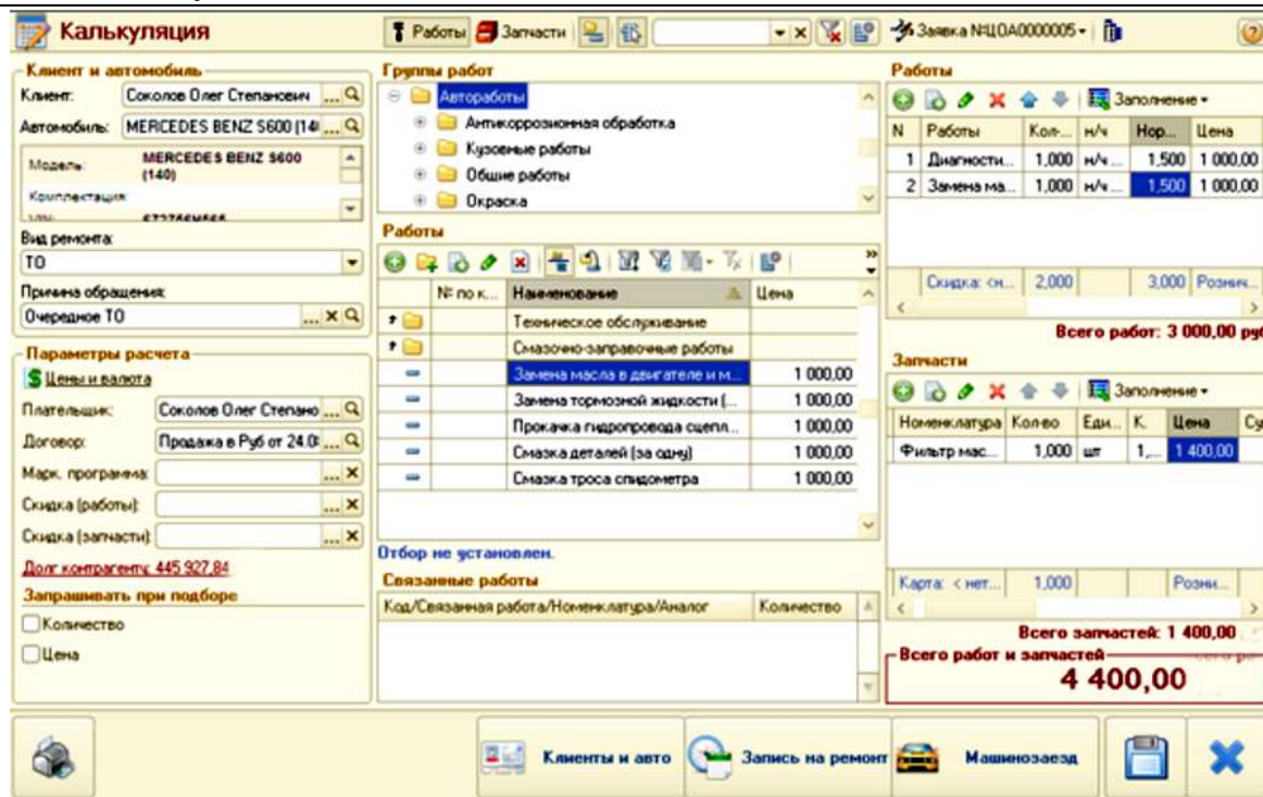
Рис. 1. Вікно програмного пакету «Альфа-Авто» у режимі «Калькуляція ремонту автомобіля»
