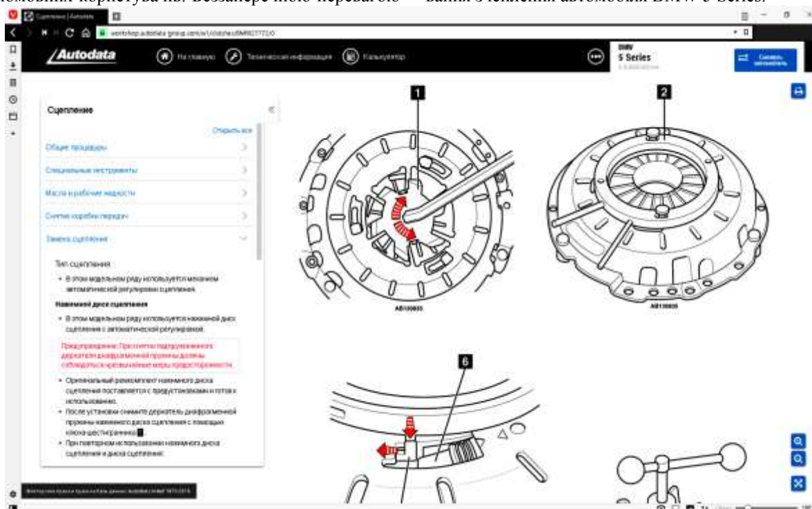
Рис. 2. Вікно програми «AutoData» у режимі «Силовий агрегат» («Зчеплення»)
