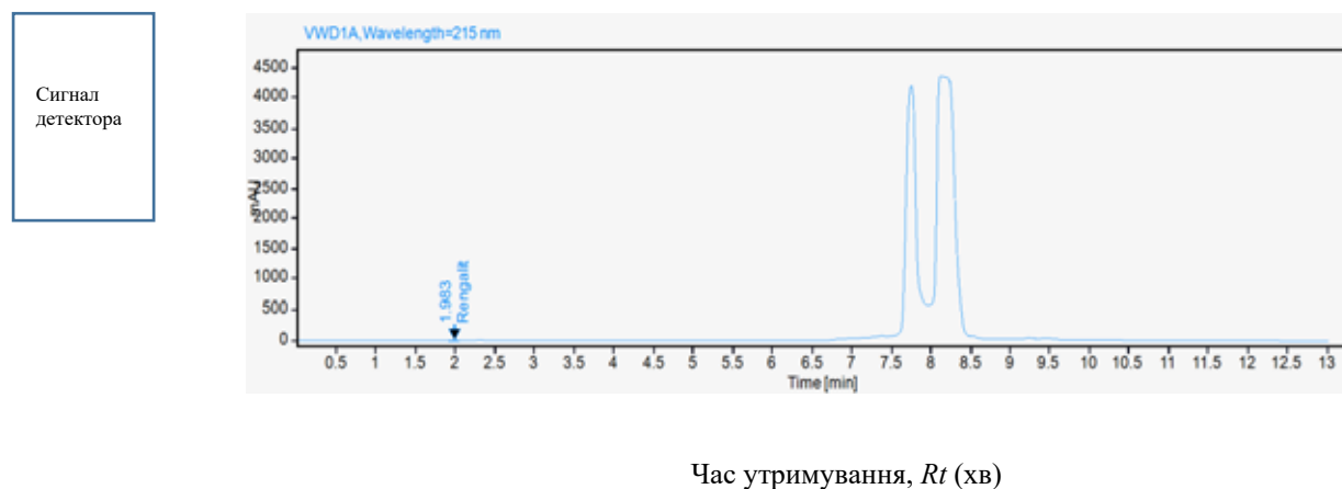
Рис. 3. Хроматограма досліджуваного зразка метамізолу натрію субстанції з домішкою ронгаліту (метод ВЕРХ) – R_t (ронгаліт) 1,983 хв
